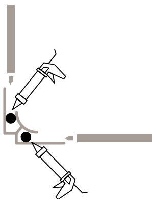
Vue de dessus profilé d'angle
